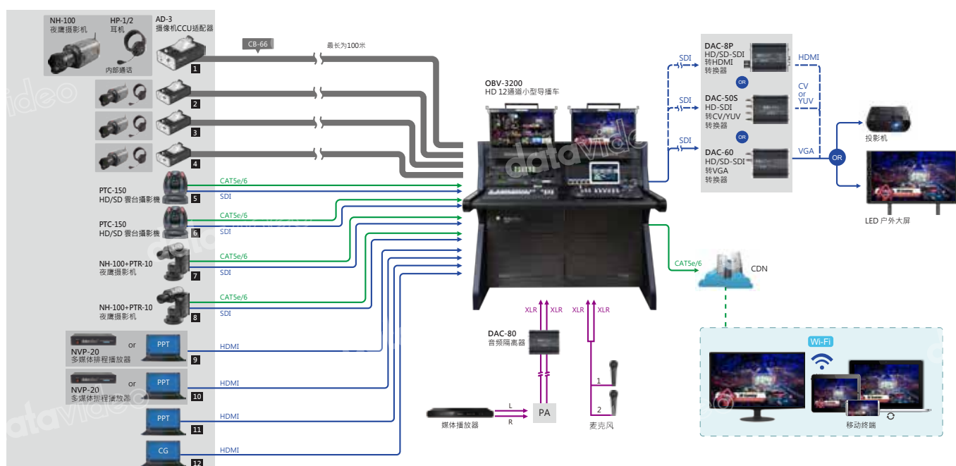
系统图
