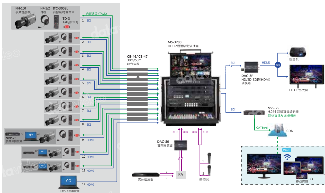
系统图
